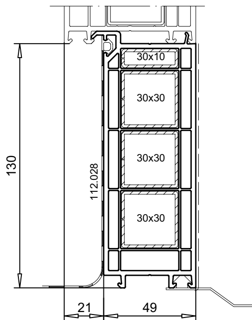
Balkonanschlussprofil 109.569 Verstärkung 113.025 / 113.020 Sondereinschlaganker 141.137
